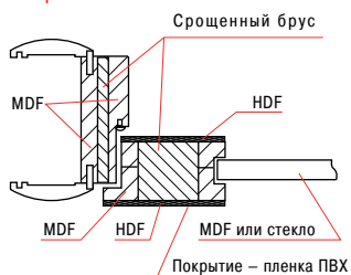
Горизонтальное сечение
